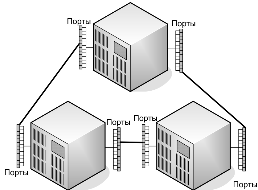
Рис. 3.2 Кольцевая схема соединения Ethernet коммутаторов
