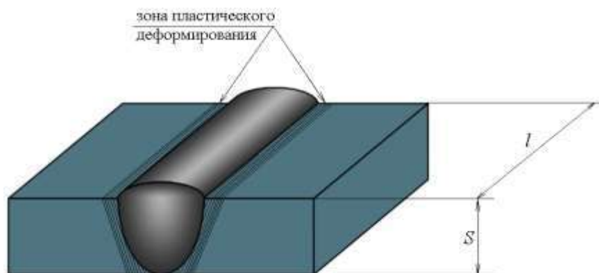
Рис. 1. Сварное соединение встык
