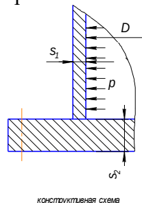
конструктивная схема
