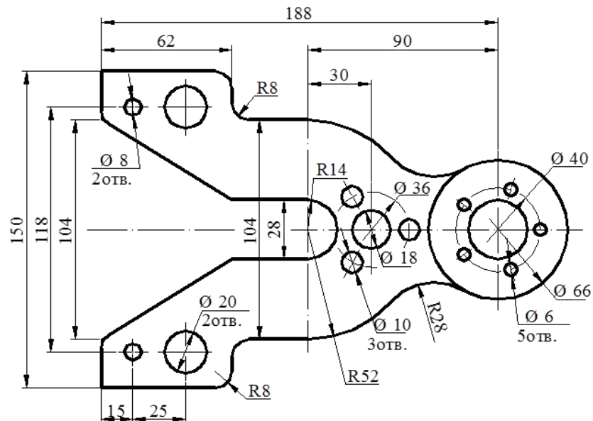
Корпус
