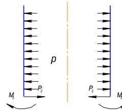
силовая схема
