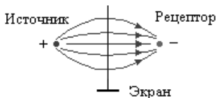
Рис. 2. Экранирование статического поля
