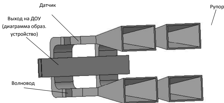
Рис. 1. Внешний вид АР для ГЗА
