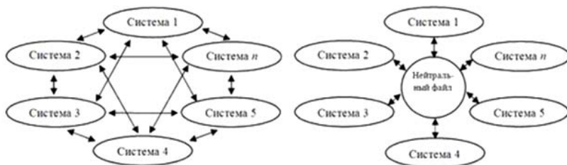
Рис. 1. Схемы обмена данными между CAD-системами
