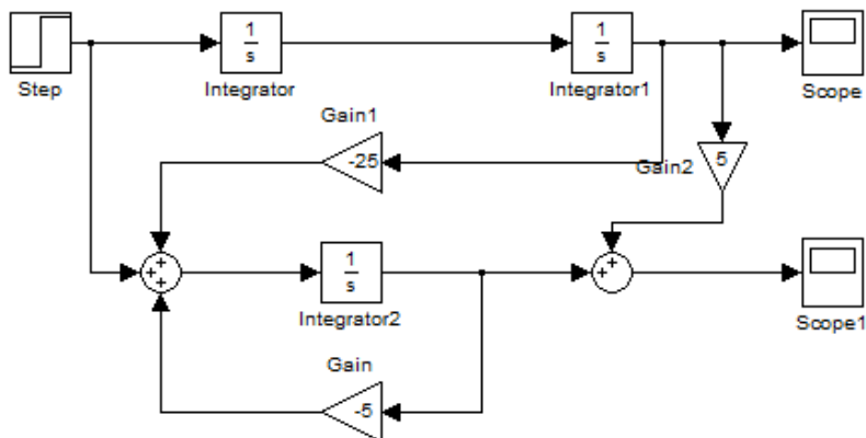
Рис. 1. Наблюдатель Льюенбергера
