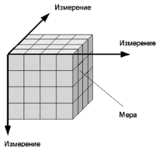
Рис. 1. Вид OLAP-куба
